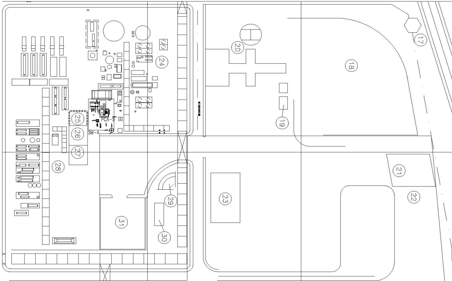
PLANTA DE AZUFRE No.2 EN EL CPG MATAPIONCHE, VER.
